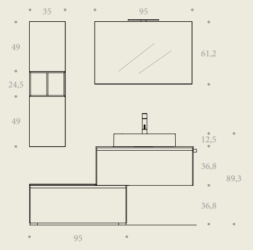
# 17. L 160,7 x P 50,5 cm (L 168,2 con sporgenza portasalviette)
