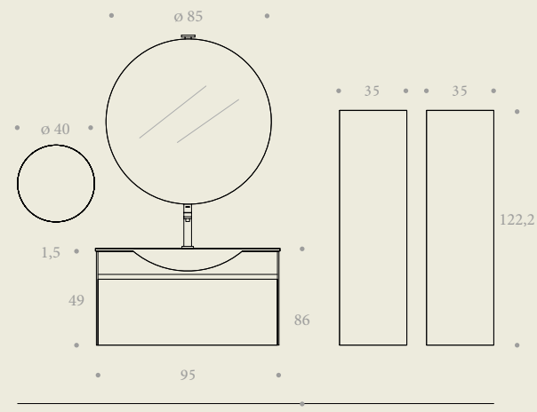
# 13. L 96 x P 37,5/44 cm + colonne L 35 x P 20,8 cm
