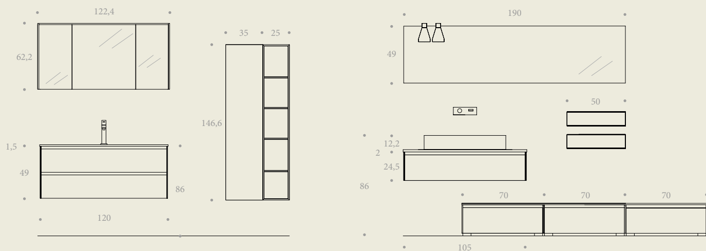
# 20. L 122,4 x P 51,5 cm + colonna L 60 x P 37 cm
