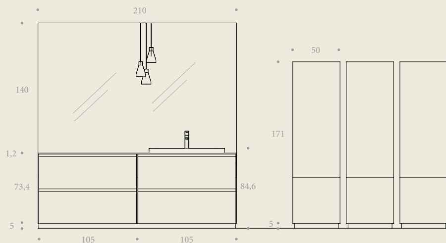
# 22. L 211 x P 50,5 cm + colonne L 50 x P 37 cm
